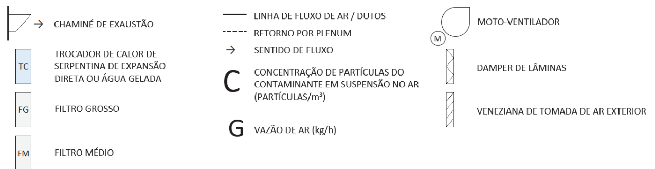
Figura 2 – Identificação dos componentes do fluxograma esquemático
